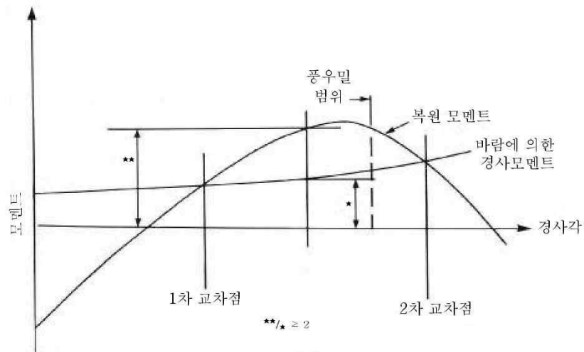
[그림 3-2] 복원모멘트 및 바람경사모멘트곡선
